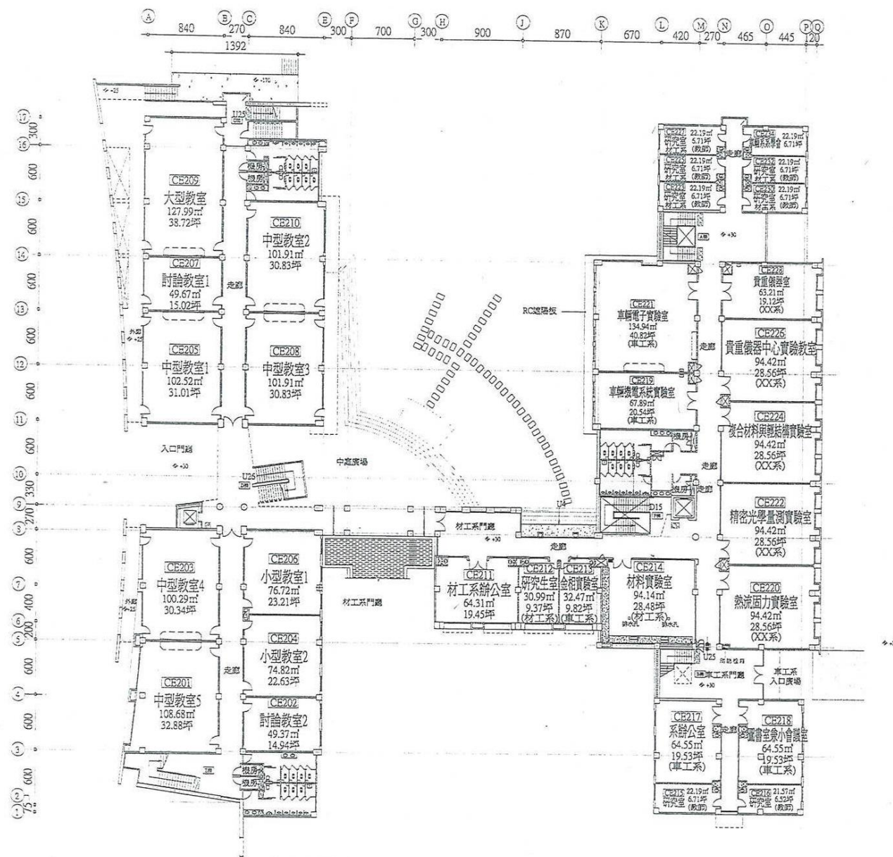
貳層平面圖
